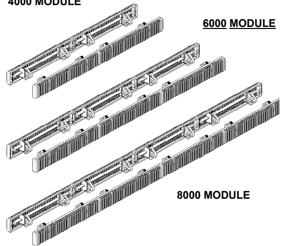
4000 MODULE
