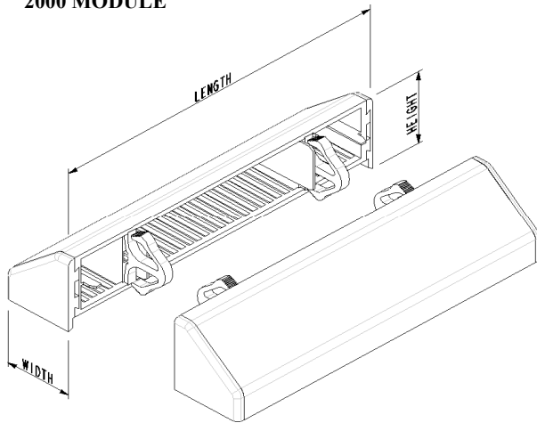
2000 MODULE
